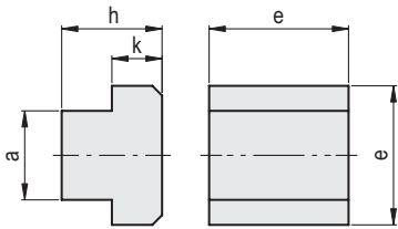
DIN 508-8 DIN 508-NI
